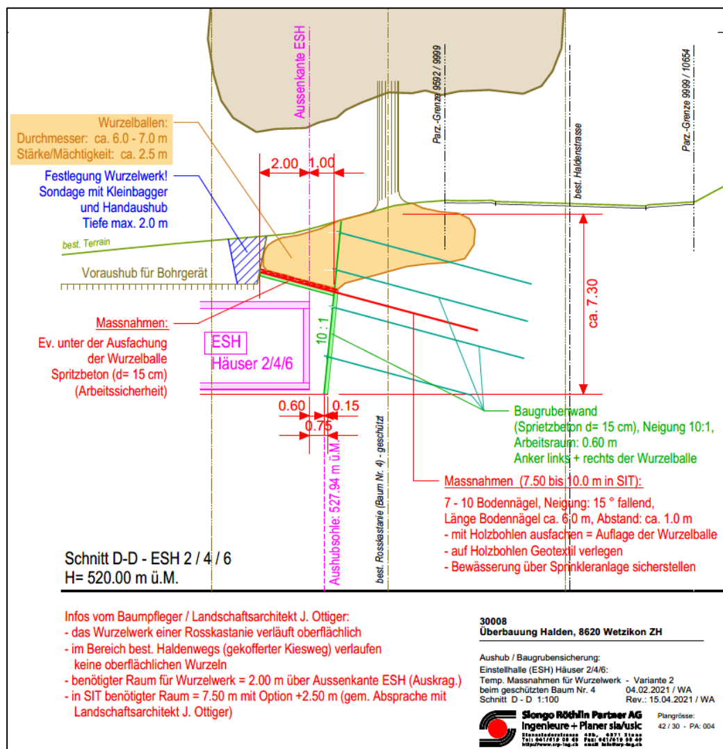
Abb. 1: Vorschlag der Bauherrschaft: mit der geplanten Abgrabung und Unterfangung kann die Rosskastanie erhalten werden.
