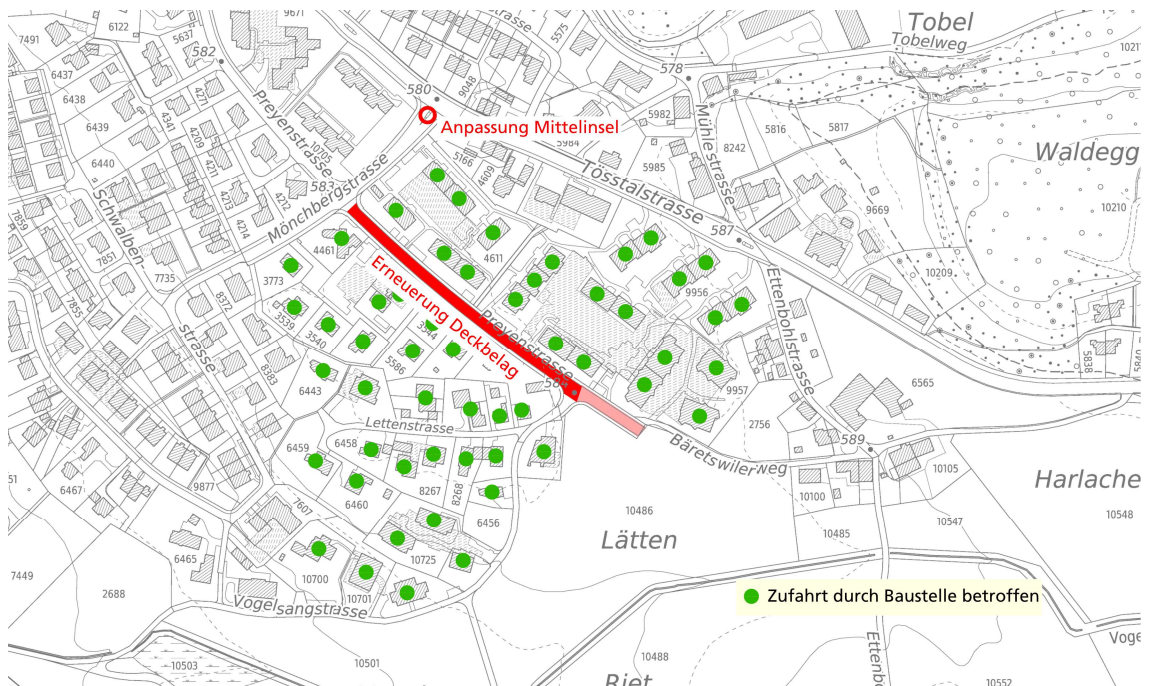
Übersichtsplan 1:5000 mit vom Bau betroffenen Liegenschaften.
