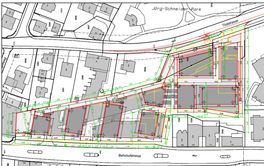
Abbildung 2: Situationsplan Bauprojekt [REDACTED], Stand 6. Januar 2021
