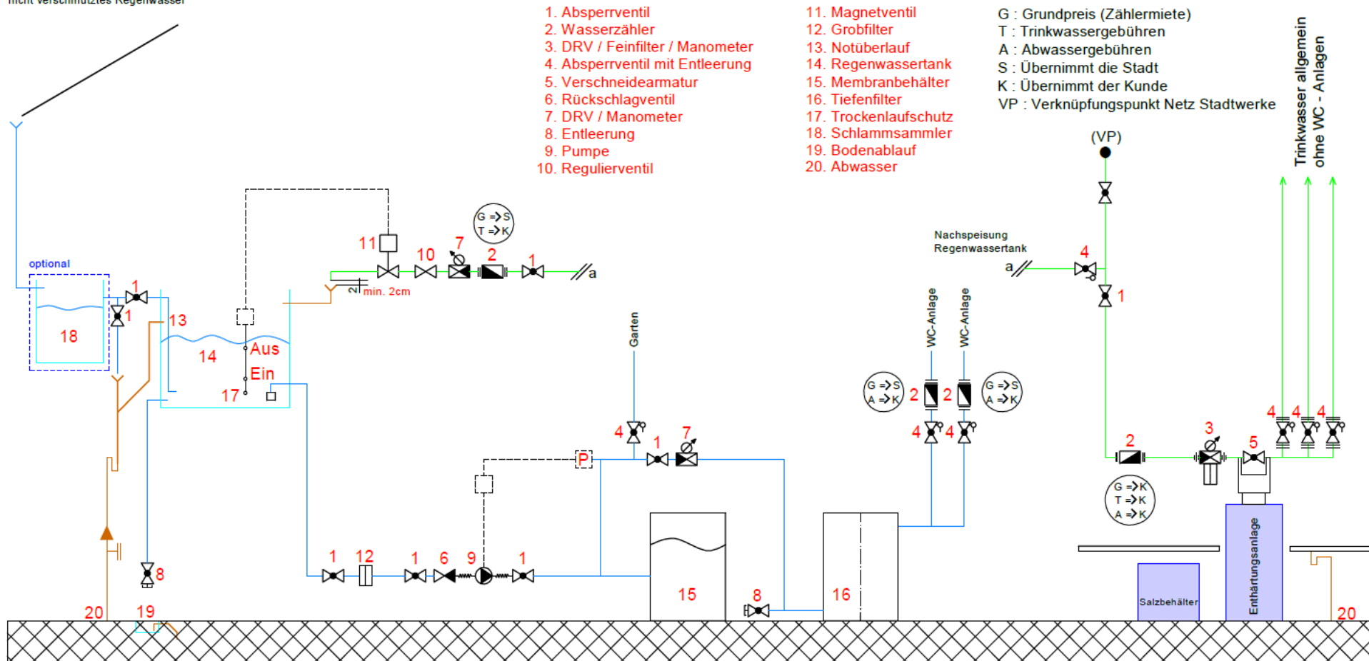
Abbildung 2 Detailschema Regenwassernutzung
