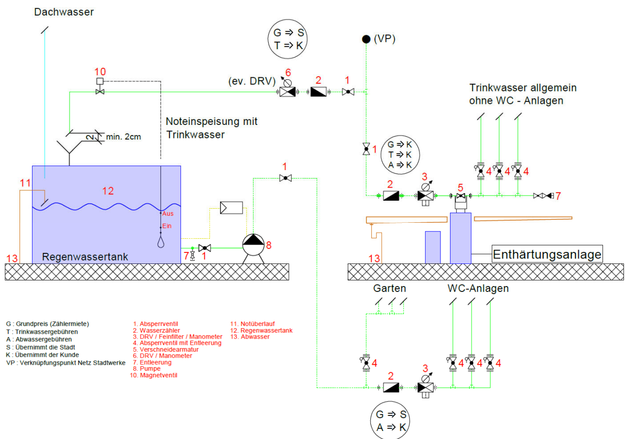
Abbildung 1 Prinzipschema Regenwassernutzung
